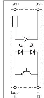
簡化電路圖
