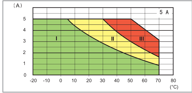
L77-2 輸出RMS電流與環境溫度 77.01.8.230.805x @ 265 V AC
