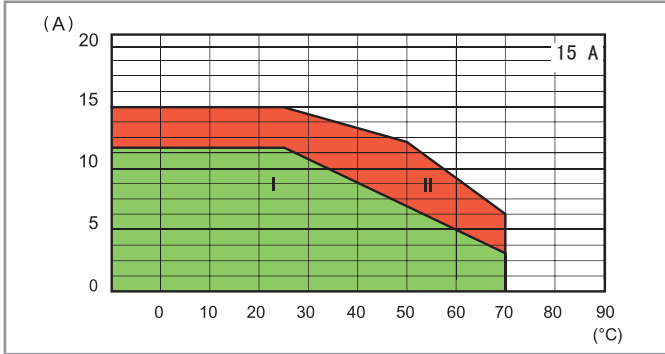
L77-12 直流電流輸出對比環境溫度 77.01.9.024.9024 @ 32 V DC
