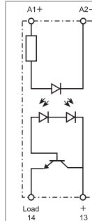
簡化電路圖
