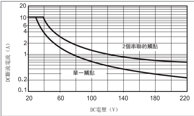
H 40.6 - 最大DC1斷流容量 類型40.62 (頁5)
