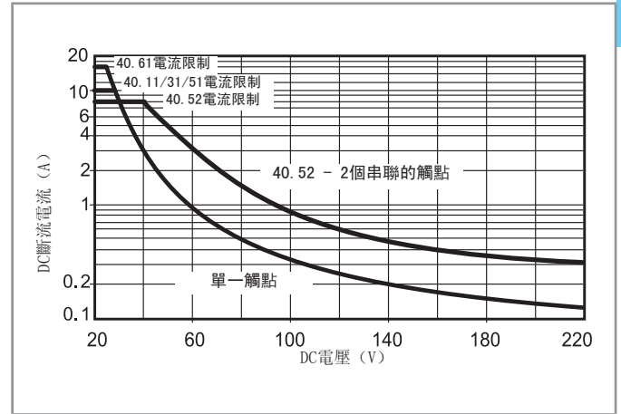
H 40.2 - 最大DC1斷流容量 類型40.31/51/52/61 (頁4) 和40.11 (頁5)
