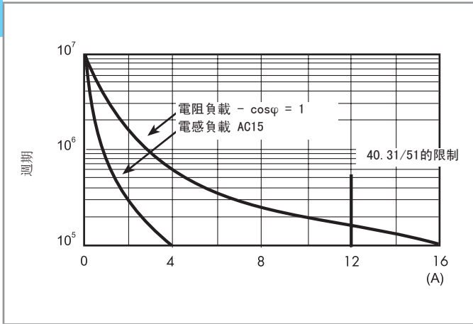
F 40.3 - 電氣壽命 (AC) 與觸點電流 類型 40.31/51/61 (頁 10)
