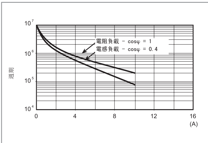
F 40.5 - 電氣壽命 (AC) 與觸點電流 類型40.11 (頁 5)
