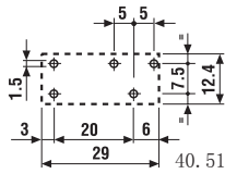
PCB銅箔側視圖 針腳長度5.3 mm，適用於PCB或插座
