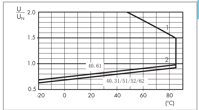
R 40 - DC線圈操作範圍與環境溫度 靈敏型線圈，類型40.31/51/52/61/62
