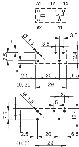
PCB銅箔側視圖 針腳長度3.5 mm只適用於PCB安裝 針腳長度5.3 mm，適用於PCB或插座 請參閱訂購訊息
