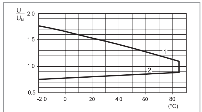
R 40 - AC線圈操作範圍與環境溫度
