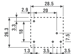
PCB銅箔側視圖 針腳長度3.5 mm，適用於 PCB或插座
