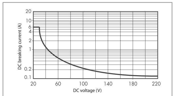
H 34 - 最大DC1斷流容量
