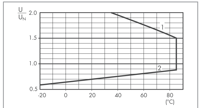
R 34 - DC 線圈操作範圍與環境溫度
